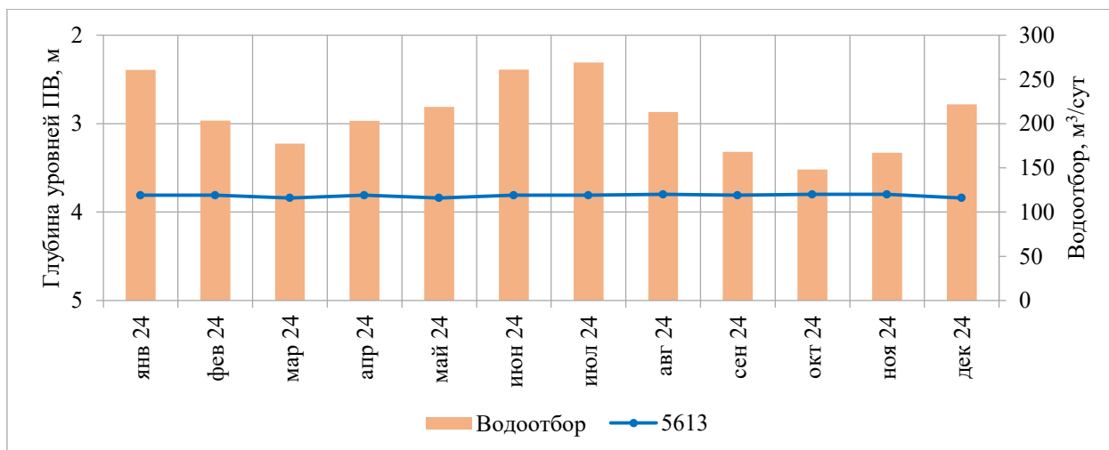
Рис. 1.29. График уровня подземных вод и водоотбора на Фронтовом водозаборе в 2024 году
