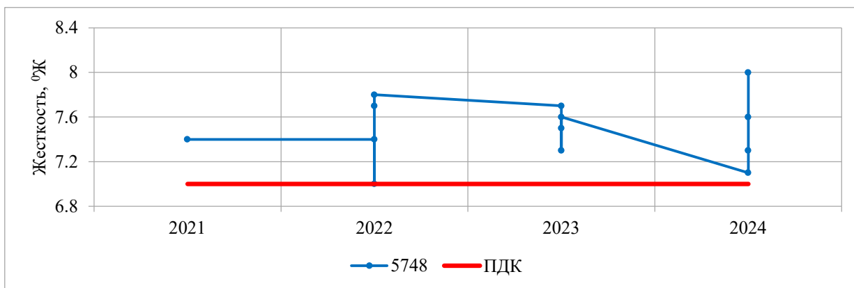
Рис. 1.72. Графики среднегодовых значений показателя жесткости общей в подземных водах на Терновском водозаборе за период наблюдений
