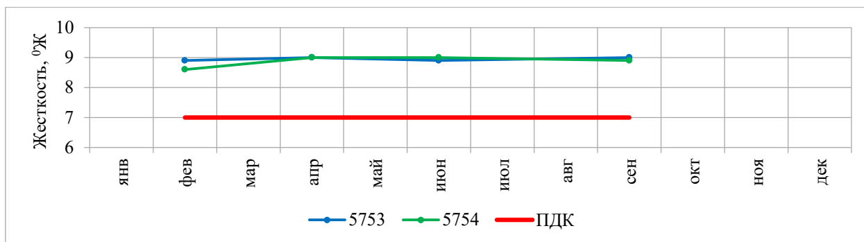
Рис. 1.67. Графики показателя жесткости общей в подземных водах на водозаборе Любимовский-1 в 2024 г.
