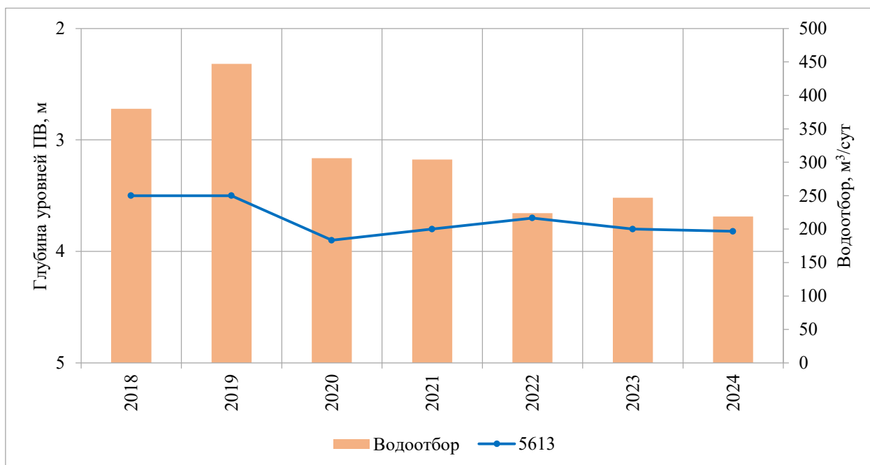
Рис. 1.30. Графики среднегодовых значений уровня подземных вод и водоотбора на Фронтовом водозаборе за период наблюдений
